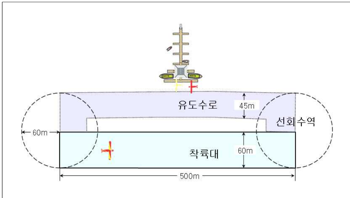
[별표 4] 수상비행장 모형도(제3장 관련)
